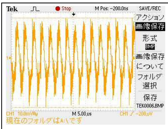
72mV p-p / 5.00µs
