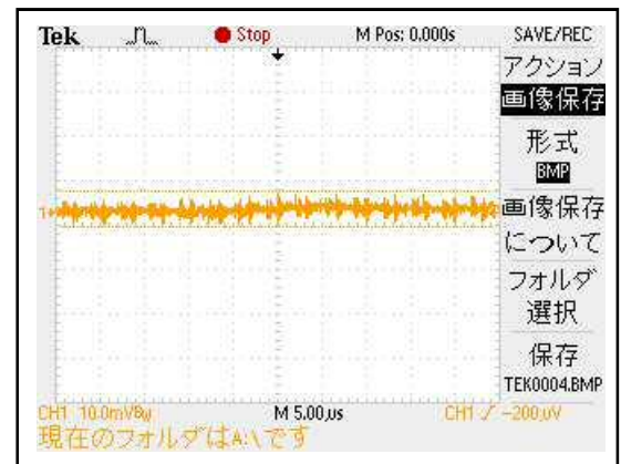
8mV p-p / 5.00µs
